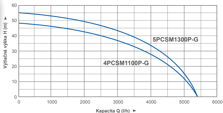
HYDRAULICKÁ KŘIVKA VÝKONU
